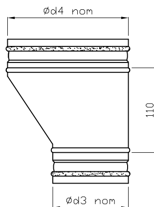
AUMENTO ECCENTRICO IN ACCIAIO MM \phi 100/160 mm ECCENTRIC ADAPTER IN STEEL MM \phi 100/160 mm
