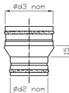
AUMENTO CONCENTRICO IN ACCIAIO MM \phi 80/100 mm CONCENTRIC ADAPTER IN STEEL MM \phi 80/100 mm
